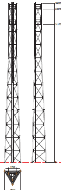
Pylône 36m
